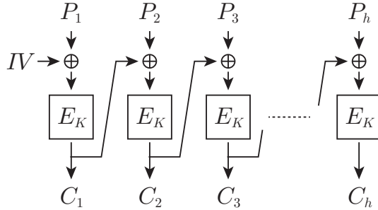
Fig. 1. CBC mode
